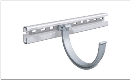
Drehhaltersystem Rinnenschiene mit Steckverbindung und Rinnendrehhalter gemäß DIN EN 1462
