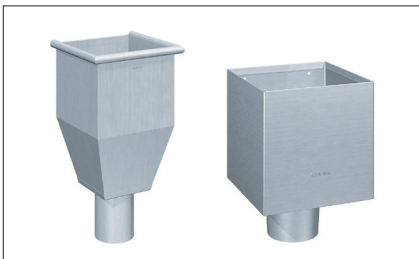
Wasserfangkasten/Wasserkubus
