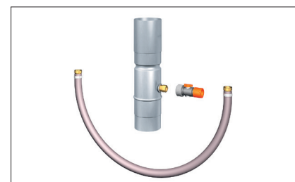
Regensammler mit GARDENA® Regulierstop (1/2 Zoll) und Verbindungsschlauch (1 Zoll) für den Direktanschluss an eine Regentonne
