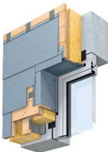
Fenstersturz/ Holz-Metall - Unterkonstruktion
