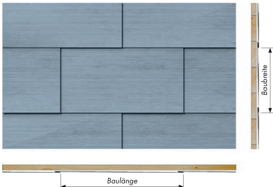
Ansicht mit Systemschnitt
