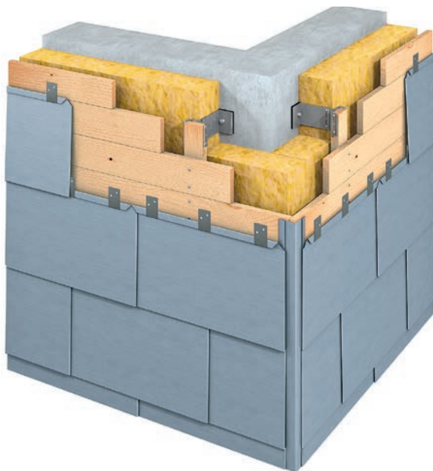
Außenecke/Holz-Metall - Unterkonstruktion (Beispielraute Achsmaß 333/600 mm)
