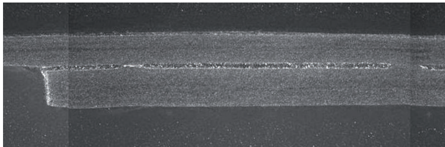
Stoffschlüssige Verbindung zwischen dem neuen bleifreien RHEINZINK-Lötzinn und dem Werkstoff RHEINZINK (Vergrößerung)
